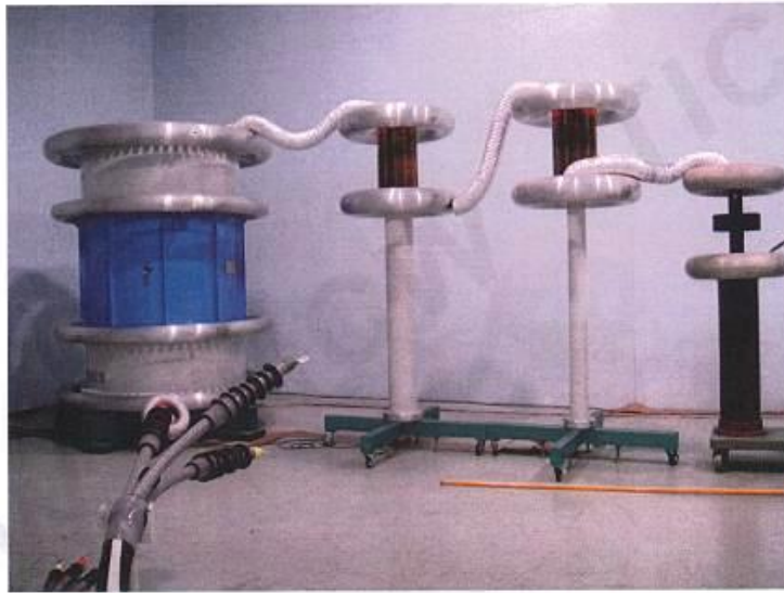
被试26/35kV三芯交联电缆冷缩式户内终端外观图
